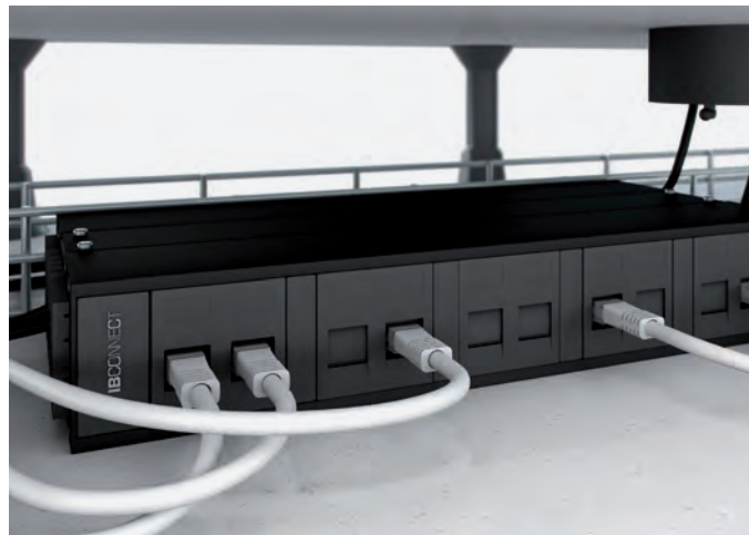
DE. RJ45-Output..
