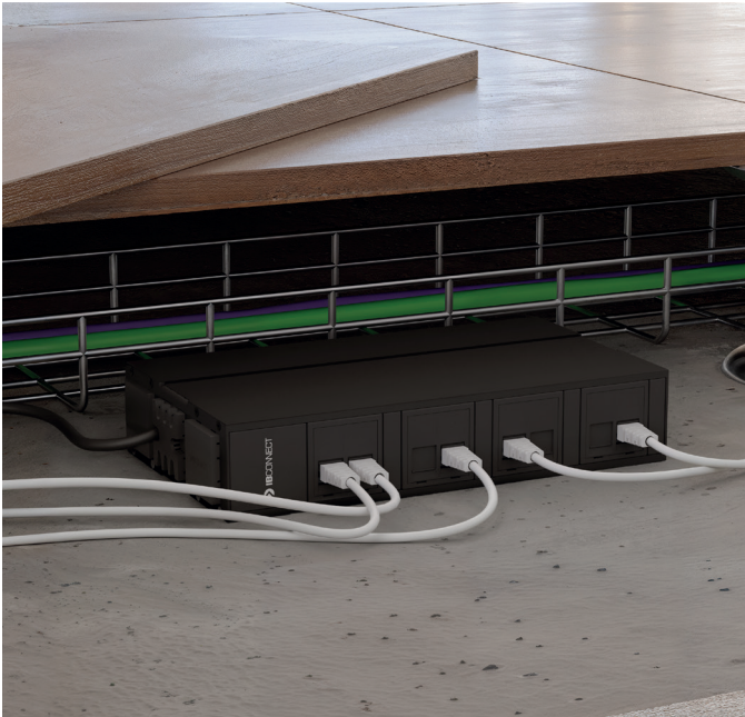
DE. RJ45-Output..
