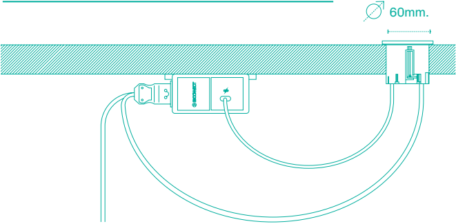
FR. Atom avec charge intelligente intègre un câble USB type C et un autre avec un connecteur rapide à l'extrémité, permettant une connexion rapide et facile au transformateur de charge (Docking).
