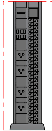
DETALLE A
